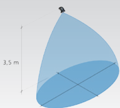
Erfassungsfeld FALCON XL 4m x 2,5m bei einer Installationshöhe von 3,5m*
