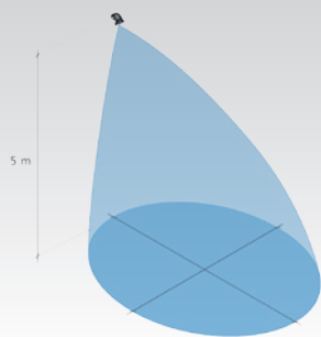
Erfassungsfeld FALCON 4m x 5m bei einer Installationshöhe von 5m*
